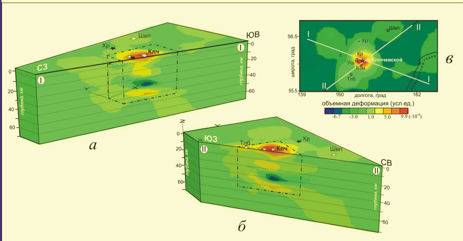
Рис. 4. Трехмерная модель объемных деформаций под КГВ. Положение профилей-сечений I (а) и II (б) показано на карте (в) распределения объемных деформаций. Пояснения географических названий в тексте.
