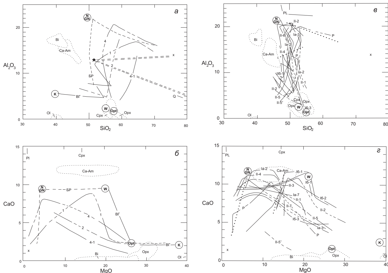
Рис. 7. Вариации составов (тренды эволюции) серий кумулатных пород в интрузивах северной зоны КНП ( а, б ) и в макрокристах расслоенности интрузива Кувалорог в южной зоне ( в, г ). Для « а » и « б » цифры на трендах соответствуют номерам интрузивов (И.Р.Т.) на рис. 1 и 2, ВГ – тренд Восточно-Геофизического интрузива, БР – тренд серии малых безрудных тел. Для « в » и « г » буквенно-цифровые индексы на трендах маркируют серии пород индивидуальных макрокристов расслоенности интрузива Кувалорог – соответственно рис. 4; р – серия пород участка Рассоха на юго-восточной оконечности интрузива, автором не изучавшейся (данные любезно предоставлены Г.В. Кувакиным). Двойные пунктиры на « а » – линии смешения исходной магмы с гранитоидными (косой крестик) и чисто кремнеземистыми (кварциты) контаминантами. Точечным пунктиром и стрелками показаны области составов главных породообразующих минералов: ОI – оливин, Оpx – ортопироксен, Сpx – клинопироксен, Pl – плагиоклаз, Са-Ам – кальциевый амфибол, Вi – биотит, в кружках – символы главных типов кумулатных пород (см. подпись к рис. 5). Пунктирами из жирных точек на « в » и « г » ограничены поля составов исходно котектических лейкогабброидов, испытавших сегрегацию вследствие селективного осаждения минералов (см. текст).
