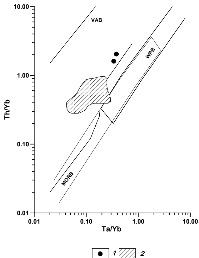
Рис. 4. Положение составов трахибазальтов на диаграмме Th/Yb – Ta/Yb: 1 – трахибазальты китильгинской толщи Валагинского хребта; 2 – трахибазальты кирганикской свиты Срединного хребта (Флеров и др., 2001 и настоящая работа). Поля базальтов различных геодинамических обстановок (Pearce, 1982): MORB – базальтов срединно-океанических хребтов; WPB – внутриплитных структур; VAB – островных дуг и активно-континентальных окраин.
