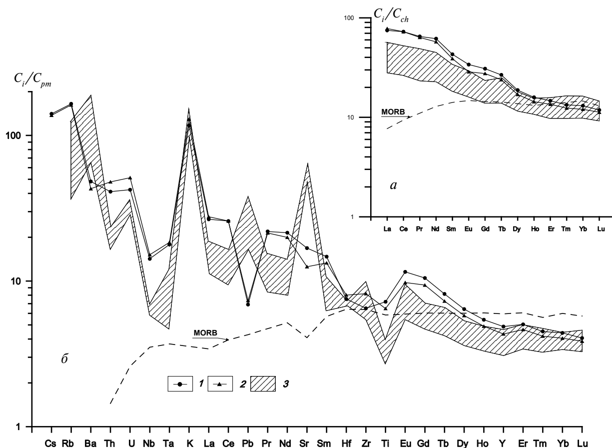
Рис. 3. Распределение редкоземельных (а) и редких (б) элементов в позднемиловых-палеогеновых калиевых породах Центральной Камчатки: 1-2 – трахибазальты китильгинской толщи Валагинского хребта: 1 – обр. 10189, 2 – обр. 10189а; 3 – трахибазальты кирганикской свиты Срединного хребта (Флеров и др., 2001 и наст. работа). Содержания некогерентных элементов в породах нормированы по примитивной мантии (pm) (Sun, McDonough, 1989) и хондриту (ch) (Pallister, Knight, 1981), состав MORB по (Sun, McDonough, 1989).
