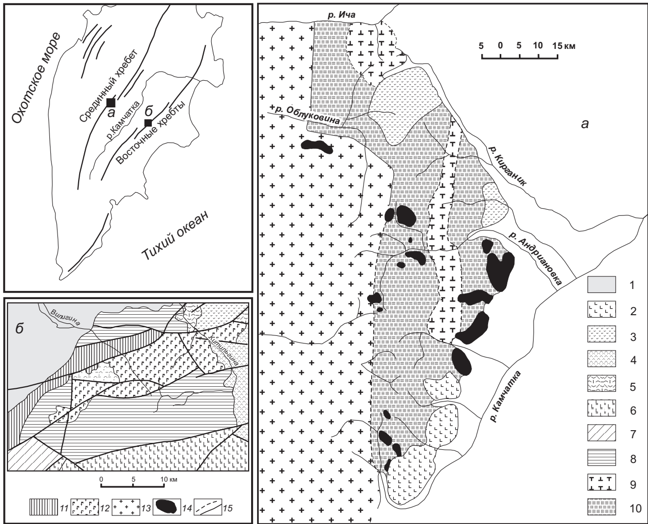
Рис. 1. Схема размещения позднемеоловых-палеогеновых калиевых вулканоплутонических комплексов на территории Центральной Камчатки (Карта ..., 1999; Флеров и др., 2001). 1 – четвертичные отложения; 2 – нижнечетвертичные базальты; 3 – неогеновые вулканогенные образования; 4 – миоценовые осадочные и вулканогенно-осадочные отложения кавранской серии; 5 – олигоцен-миоценовые осадочные и вулканогенно-осадочные отложения тюшевской серии; 6 – палеоцен-эоценовые вулканогенные и осадочные образования ветловской свиты; 7 – осадочные отложения вахвинской свиты; 8 – осадочные и вулканогенно-осадочные отложения хапицкой свиты; 9 – позднемеоловые-палеогеновые вулканыты кирганикской свиты; 10 – верхнемеловые вулканогенно-осадочные породы ирунейской свиты; 11-12 – китильгинская толща: 11 – осадочные и вулканогенно-осадочные отложения, 12 – вулканогенные и вулканогенно-осадочные образования; 13 – метаморфизованные породы (гнейсы, кристаллические сланцы) Срединного массива; 14 – массивы интрузивного комплекса; 15 – разрывные нарушения.
