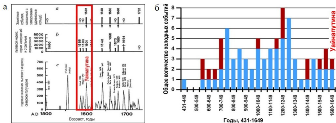
Рис. 2. «Морозные» кольца в соснах на западе США (Сьерра-Невада) и связь с крупными извержениями вулканов в глобальном масштабе [8] (а); «холодные» события, отмеченные в летописях ирландских монахов [9] (б).
