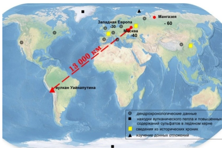
Рис. 1. Следы извержения вулкана Уайнапутина в различных районах Земли.
