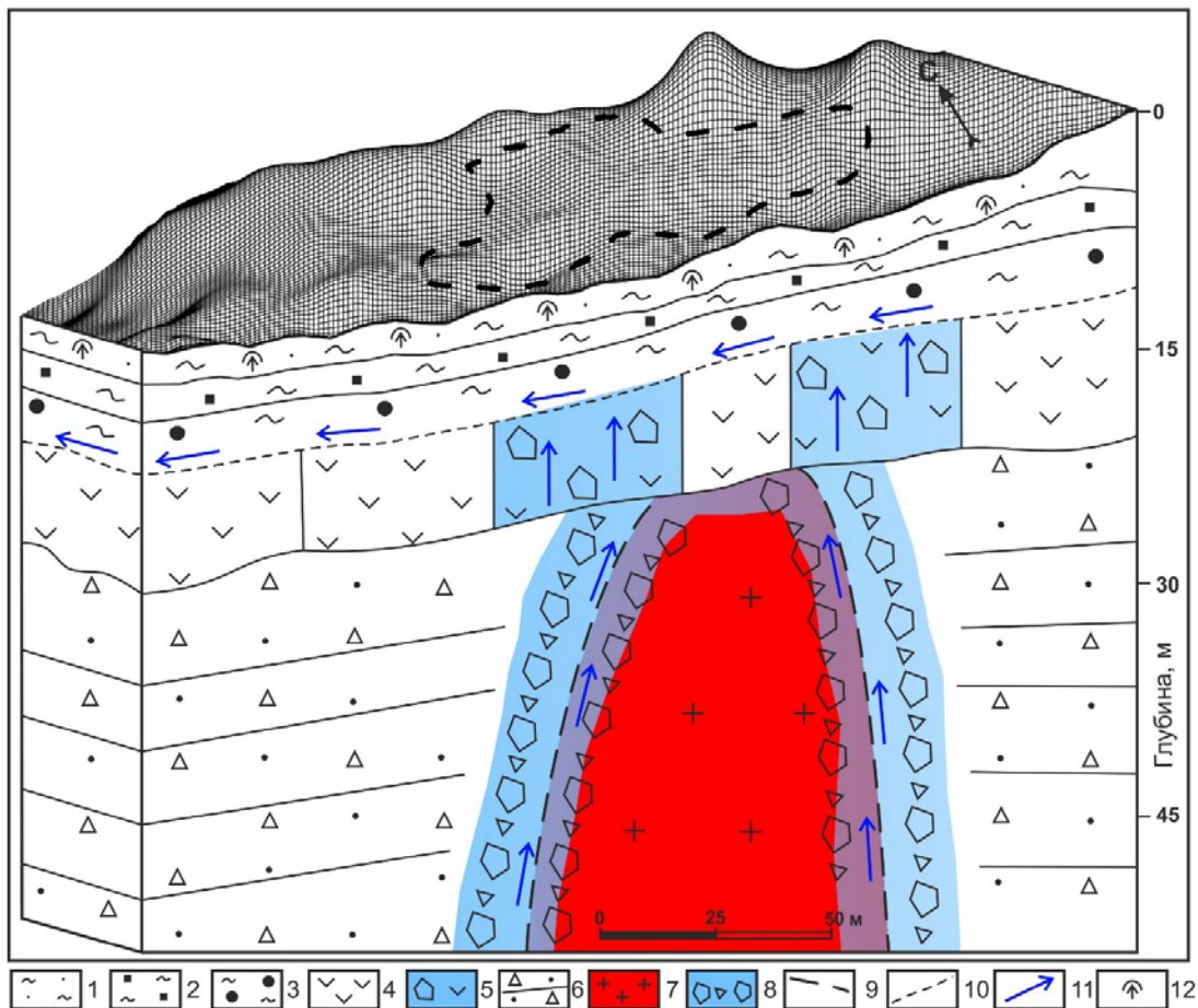
Рисунок 10. Концептуальная модель структуры зоны разгрузки парогидротерм в районе Восточно-Паужетского термального поля [Феофилактов и др., 2017]. 1 – горизонт гидротермальных глин зоны сернокислотного выщелачивания; 2 – горизонт тугопластичных влагонасыщенных глин; 3 – горизонт “сухих” глин, включающий слои с минеральными рудными ассоциациями; 4 – лавы андезитов; 5 – то же, интенсивно трещиноватые и брекчированные; 6 – туфы и туффиты верхнепаужетской подсвиты; 7 – субинтрузивные породы; 8 – брекчии в эндо-экзоконтактной зоне субинтрузивного тела; 9 – условная граница апикальной части субинтрузивного тела; 10 – подошва толщи гидротермальных глин – зона растекания смешанных термальных вод; 11 – восходящие газо-водные флюиды; 12 – зона интенсивного испарения влаги. В плане на рельеф дневной поверхности наложен условный контур неоднородности, отраженной в различных физических полях и совпадающей с наиболее прогретой частью термального поля.
