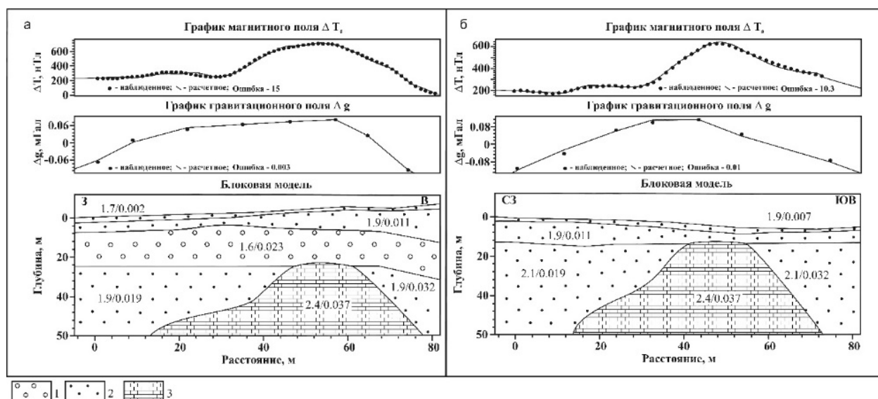
Рисунок 9. Модель структуры Восточно-Паужетского термального поля, построенная на основании гравиразведочных, магниторазведочных и литологических данных по профилям: а – по меридиональному, б – по широтному. 1 – группа блоков с плотностью 1.6 \text{ г/см}^3 , 2 – то же, 1.7-2.1 \text{ г/см}^3 , 3 – то же, 2.4 \text{ г/см}^3 [Феофилактов и др., 2017]. Цифрами на схеме отмечены средние значения плотности и магнитной восприимчивости (в знаменателе) для каждого блока.
