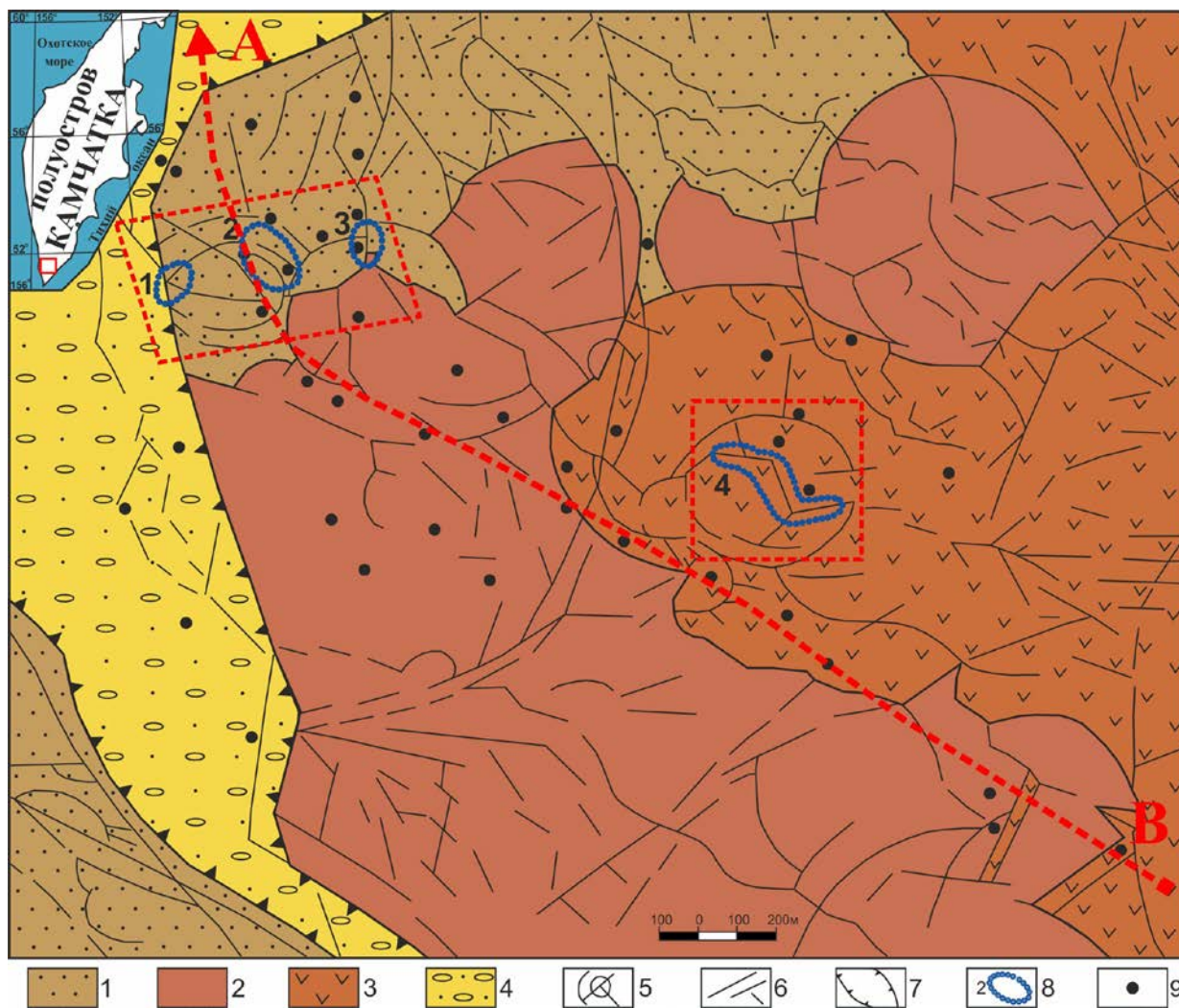
Рисунок 2. Схематическая геологическая карта Паужетской гидротермальной системы с дополнениями [Структура ..., 1993]. 1 – туффиты и туфы верхнепаужетской подбиты верхней неоген -нижнечетвертичного возраста; 2 – лаво-экструзивный комплекс пород кислого состава среднечетвертичного возраста; 3 – андезиты и андезибазальты среднечетвертичного возраста; 4 – аллювиальные валунно-галечные отложения; 5 – кольцевые тектонические нарушения, оконтуривающие приподнятые блоки пород и контролирующее положение термальных полей; 6 – система линейных тектонических нарушений; 7 – Паужетский грабен верхнечетвертичного возраста; 8 – термальные поля: 1 – Южно-Паужетское, 2 – Верхне-Паужетское, 3 – Нижне-Паужетское, 4 – Восточно-Паужетское; 9 – глубокие скважины.
