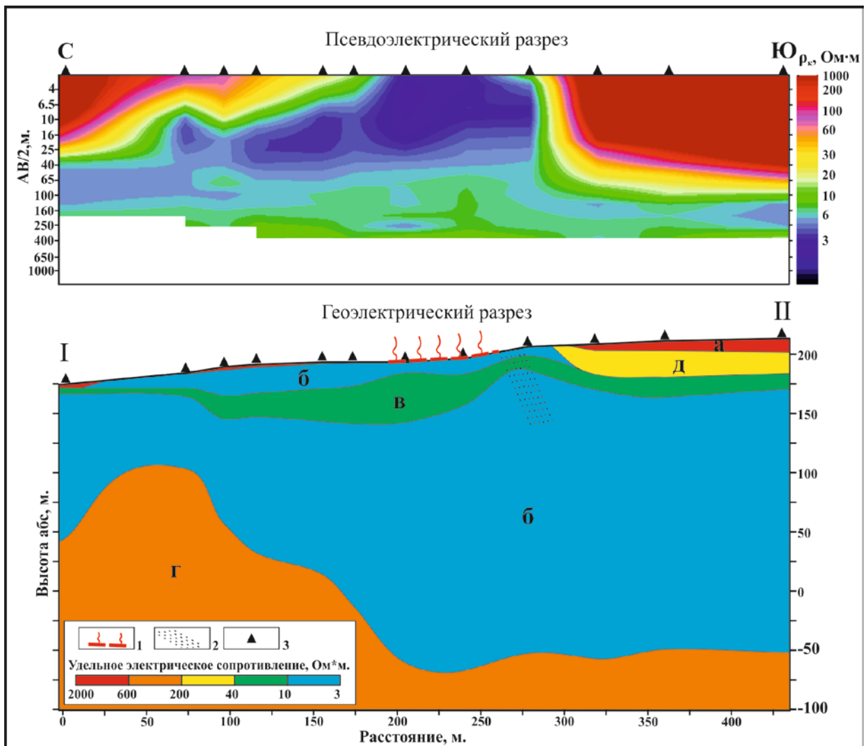
Рисунок 5. Псевдо- и геозлектрический разрезы района Верхне-Паужетского термального поля [Феофилактов и др., 2020]: а-д – слои, контрастные по удельному электрическому сопротивлению среды (см. текст). 1 – область разгрузки парогидротерм на дневной поверхности; 2 – зона нарушения сплошности среды; 3 – пункты ВЭЗ.
