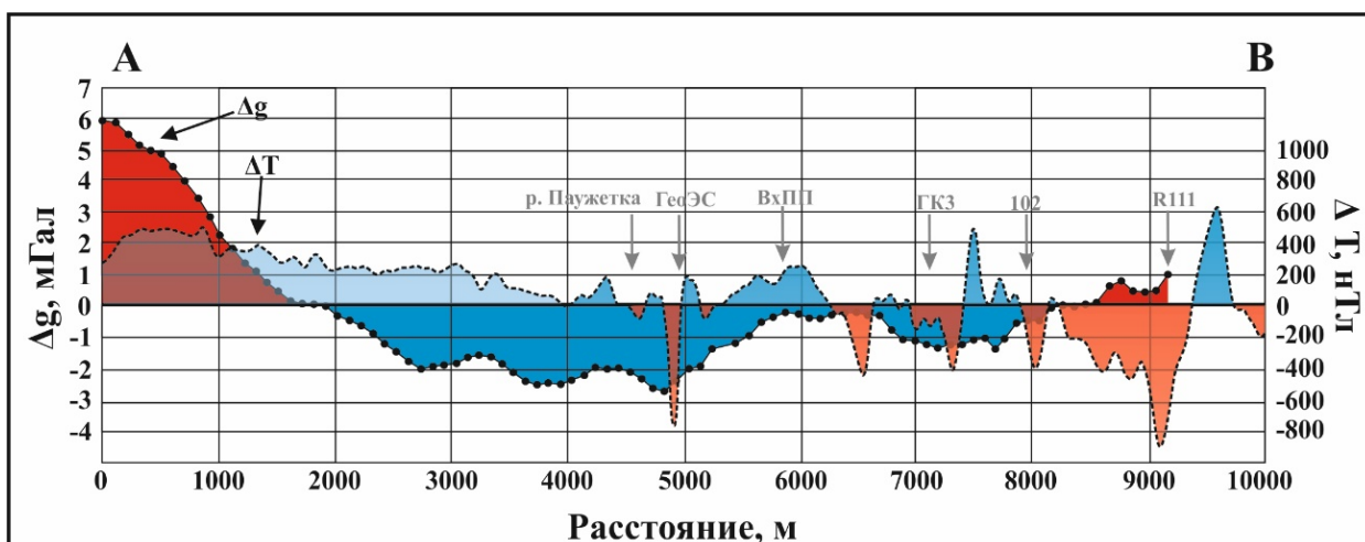
Рисунок 8. Графики распределения значений аномального магнитного поля ( \Delta T_a ) и гравитационного поля в редукции Буге ( \Delta g ) с учетом рельефа местности по профилю А - В [Феофилактов и др., 2021].
