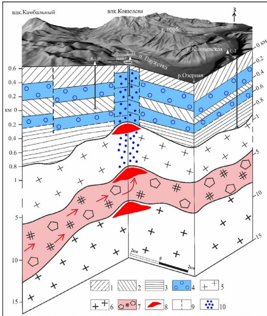
Рисунок 13. Концептуальная модель строения района Паужетской гидротермальной системы [Феофилактов и др., 2021]. 1-3 – Водоупорные горизонты в геологической структуре гидротермальной системы: 1 – верхний, представленный валунно-галечными аллювиальными отложениями Озерновского и Паужетского грабенных (в правой части модели), а также туффидами верхнепаужетской подсвиты и лавами Камбального вулканического хребта; 2 – средний, включающий магматические породы Ключевского комплекса и голыгинские игнимбриты района геотермального месторождения; 3 – нижний, отвечающий толще анавагйских песчаников. 4 – водовмещающий комплекс пород, состоящий из туфов паужетской свиты (верхний горизонт) и туфобрекчий аллейской серии (нижний горизонт); 5 – меловой фундамент; 6 – кристаллический фундамент; 7 – область разуплотненных горных пород в кровле кристаллического фундамента (подошве мелового фундамента), соответствующая предполагаемой зоне повышенной проводимости геотермального флюида; 8 – крупные интрузивные комплексы; 9 – субвертикальные разрывные нарушения; 10 – поток геотермального флюида, приуроченный к выступам мелового и кристаллического фундаментов и (или) к крупным интрузивным комплексам. Стрелками показано направление движения глубинного флюида - из-под основания Камбального хребта.
