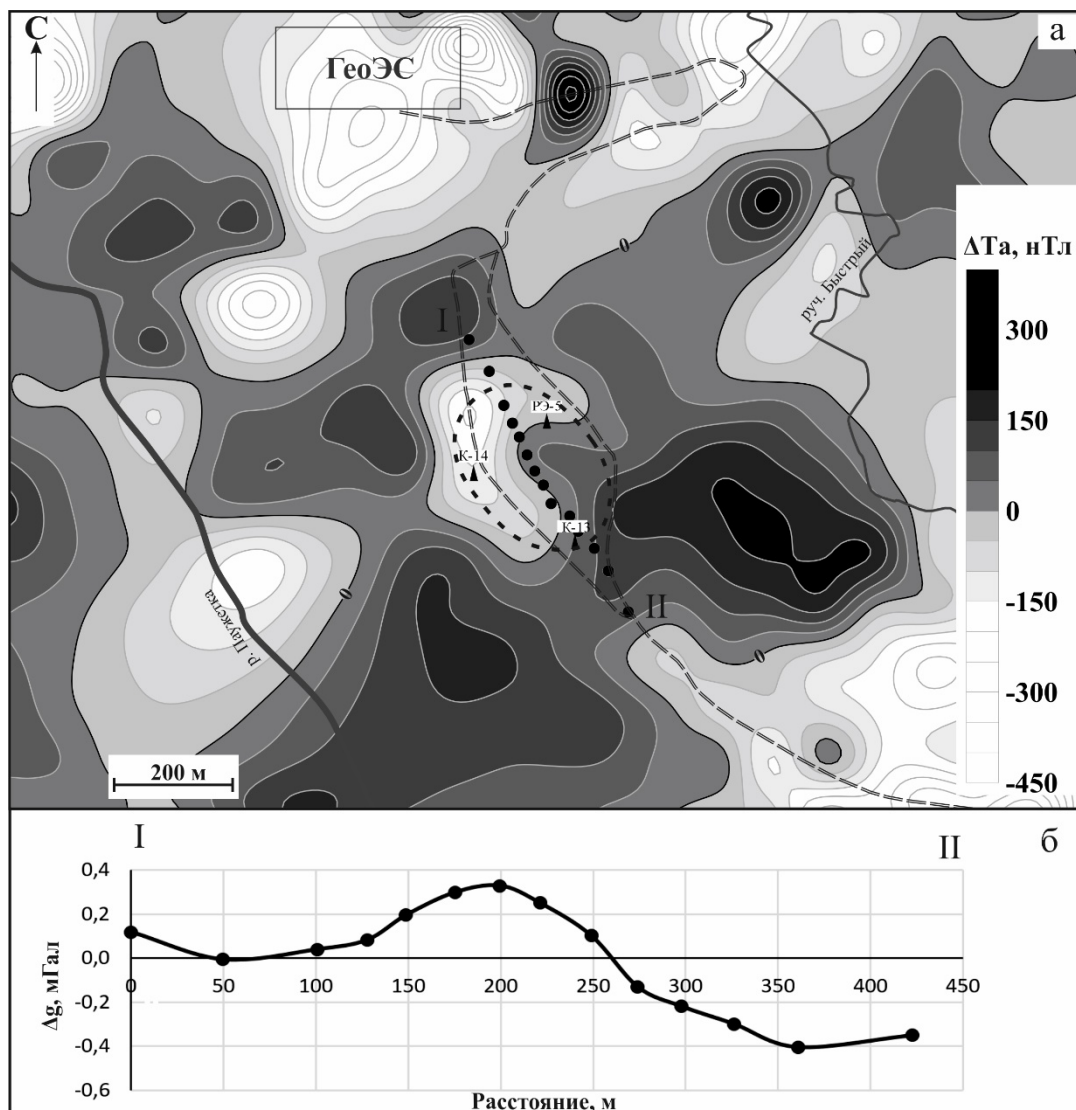
Рисунок 6. Схема распределения значений аномального магнитного \Delta T_a в центральной части Паужетского геотермального месторождения (а) и график распределения значений аномального гравитационного поля в редукции Буге ( \Delta g ) по профилю (б) [Феофилактов и др., 2020]. Пунктиром выделен район Верхне-Паужетского термального поля.
