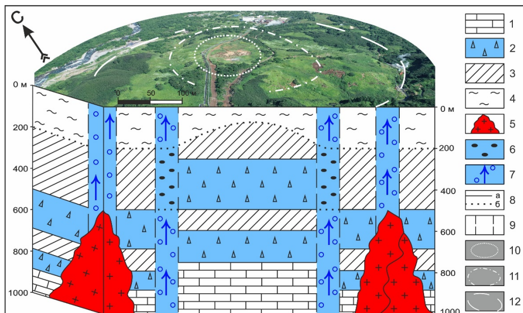
Рисунок 12. Концептуальная модель структуры района Верхне-Паужетского термального поля Паужетской гидротермальной системы [Феофилактос и др., 2020]. Использовано фото М.С. Чернова. 1 – фундамент структуры: вулканомиктовые песчаники; 2 – водовмещающие толщи пород: нижняя – агломератовые туфы, верхняя – псефитовые туфы; 3 – водоупорные горизонты: нижний – игнимбриты, верхний – туффиты; 4 – аргиллизированные породы; 5 – субвулканические интрузии; 6 – кварцадуляровые метасоматиты; 7 – зоны подъема и разгрузки газоводных флюидов и парогидротерм; 8 – литологические (а) и метасоматические (б) границы; 9 – зоны разрывных тектонических нарушений; 10 – границы термального поля; 11 – осевая линия зоны тектонических нарушений, оконтуривающей центральный приподнятый блок; 12 – условные границы тектоно-магматического поднятия.
