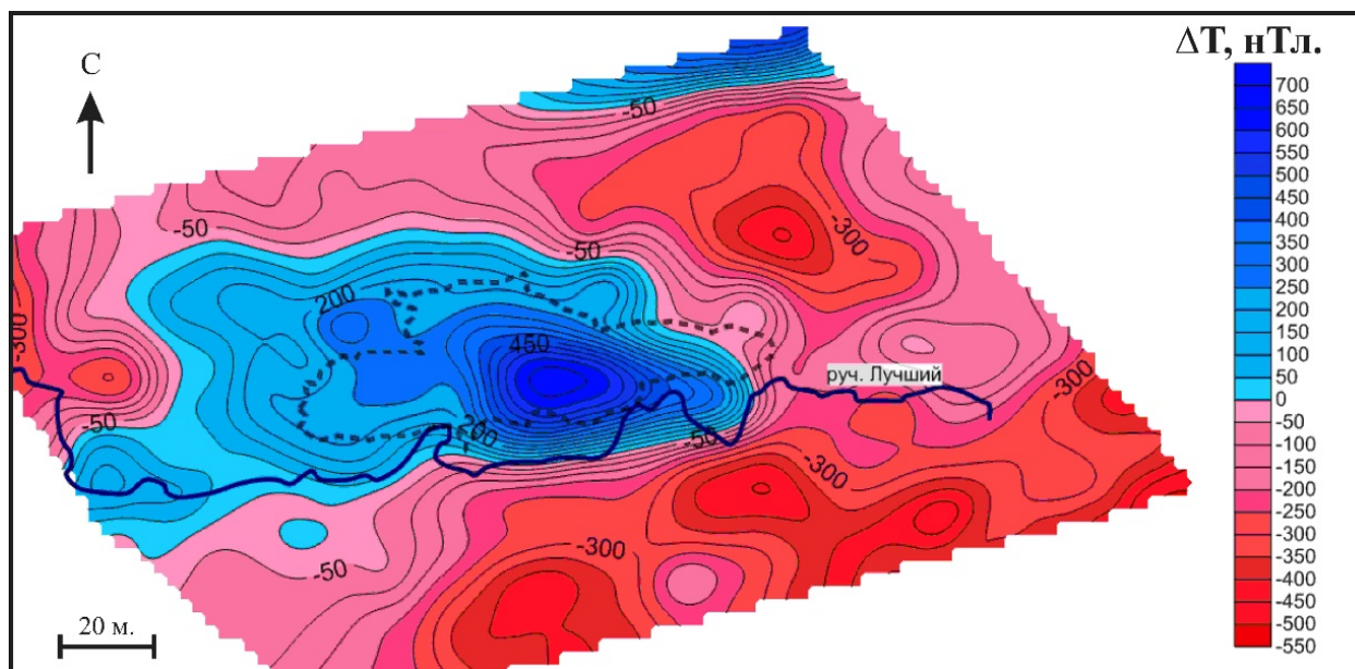
Рисунок 4. Карта распределения значений аномального магнитного поля \Delta T_a для Восточно-Паужетского термального поля [Феофилактов и др., 2017].
