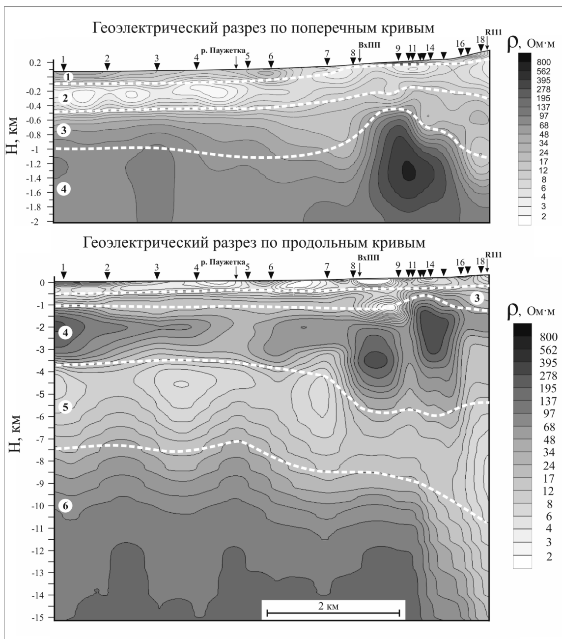
Рисунок 7. Геоэлектрический разрез района Паужетской гидротермальной системы по данным МТЗ и АМТЗ [Феофилактов и др., 2021].
