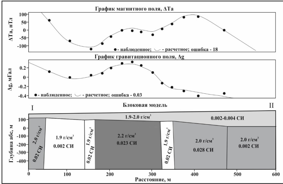
Рисунок 11. Блоковая модель строения района Верхне-Паужетского термального поля по грави-магнитным данным [Феофилактов и др., 2020].
