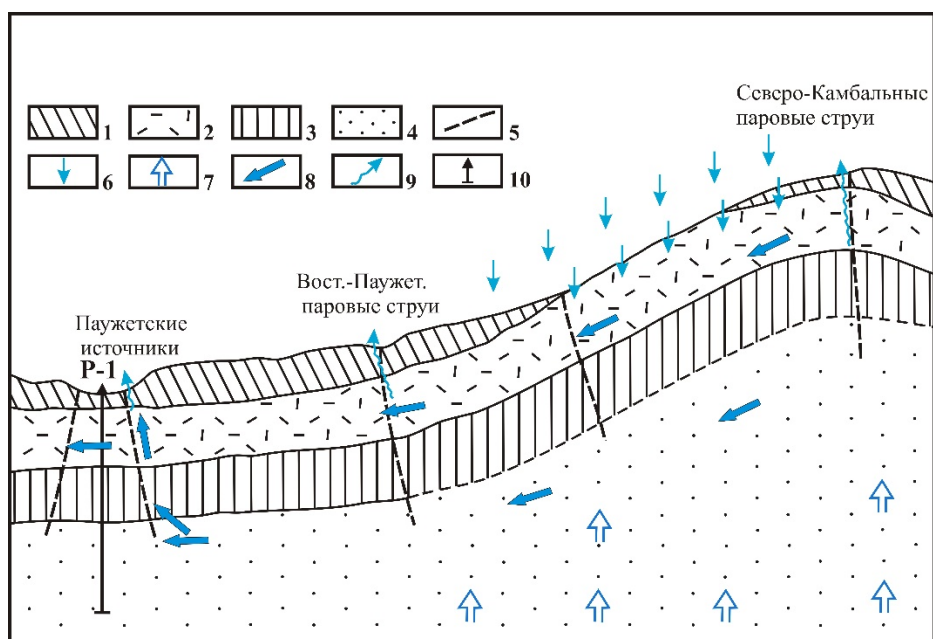
Рисунок 1. Концептуальная схема формирования и разгрузки Паужетских гидротерм [Паужетские..., 1965]. 1 – алевропелитовый чехол; 2 – псефитовые туфы; 3 – спекшиеся туфы; 4 – туфопесчаники; 5 – разломы; 6 – инфильтрационные воды; 7 – эндогенный пар; 8 – высокотермальные воды; 9 – паровые струи; 10 – скважины.
