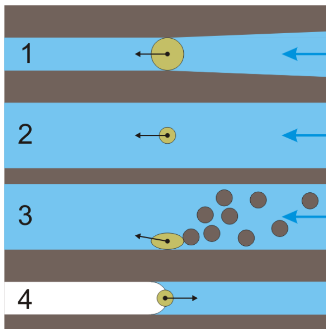
Рис. Иллюстрация механизмов срыва частиц. Цифры соответствуют номерам подзаголовков в тексте.
